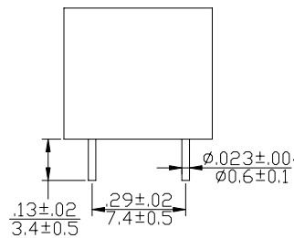
CUT: PIN2,6,7
